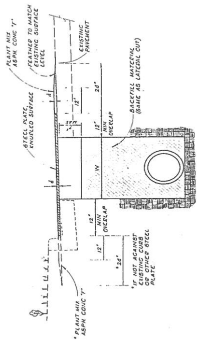
LONGITUDINAL CUT
