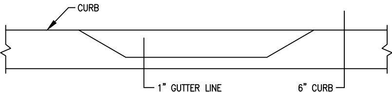
SECTION A-A N.T.S.
